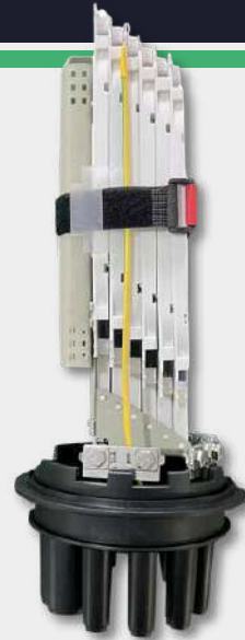
CIERRE DE EMPALME TIPO DOMO 144H
