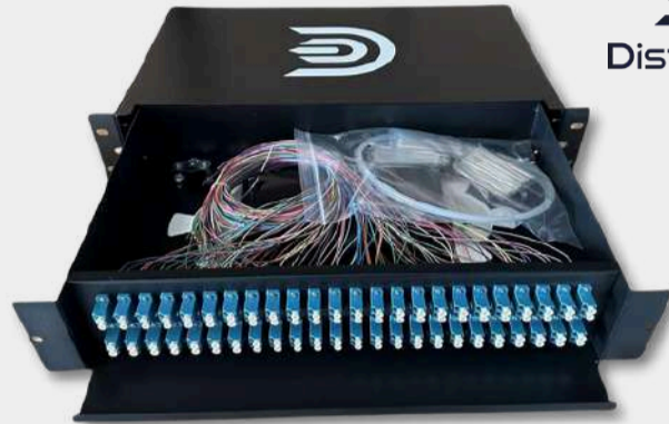
ODF- 96 puertos con lc/upc pigtails y adaptadores
